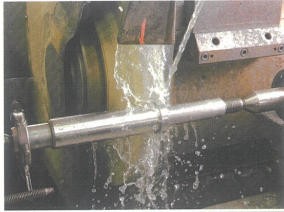
円筒研削
