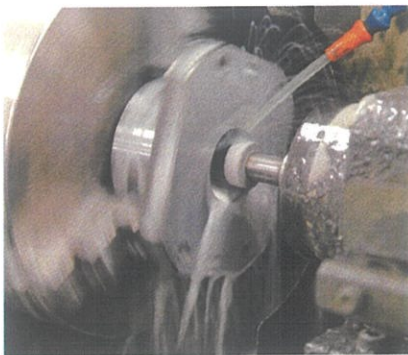
内面研削
